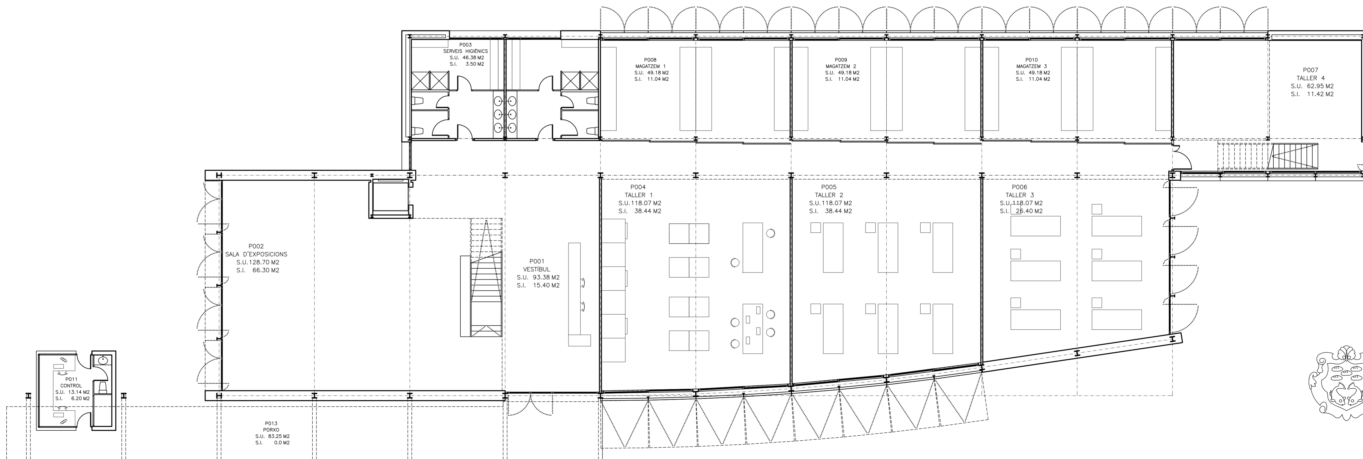
DISTRIBUCIÓ PLANTA BAIXA (ACCÉS)
