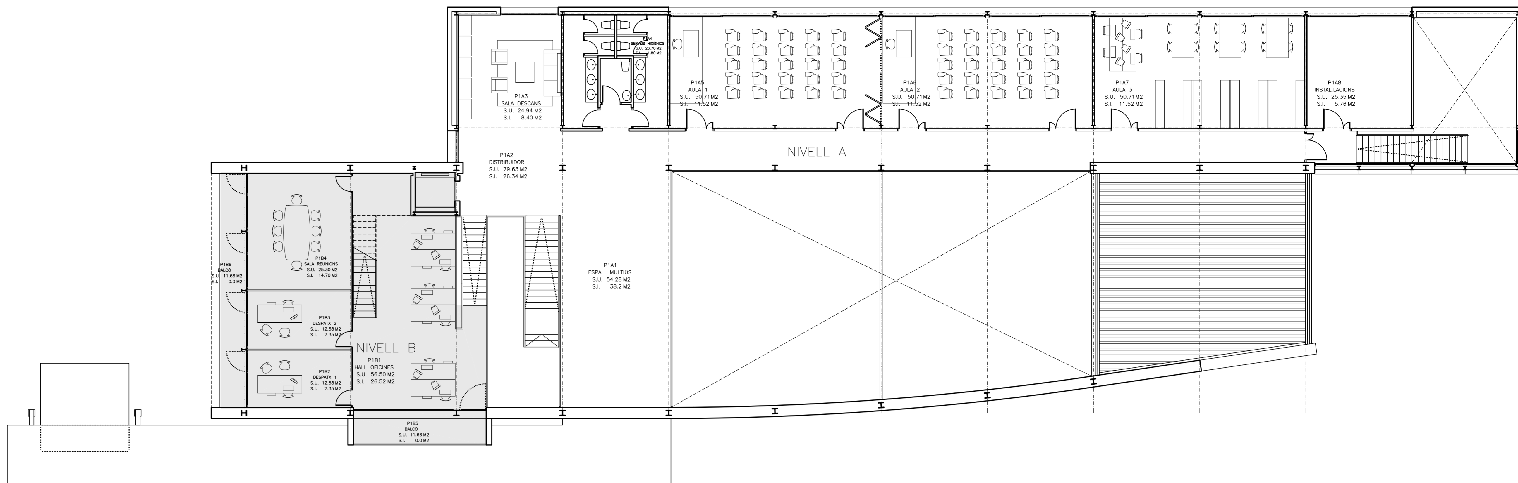
DISTRIBUCIÓ PLANTA 1 (NIVELL A i B)
